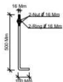
DET. Anchor Scale 1 : -
