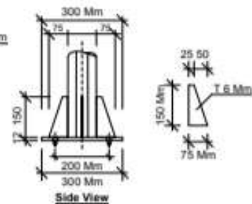
DET. Anchor Scale 1 : -
