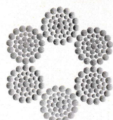
6xSeS(37)+IWRC
