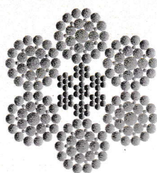
6xFi(29)+IWRC
