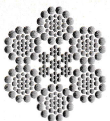
6xWS(31)+IWRC
