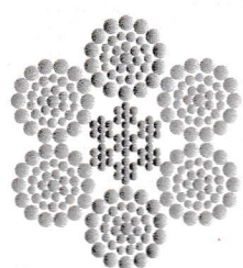
6xWS(36)+IWRC
