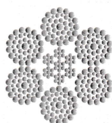
6xWS(41)+IWRC
