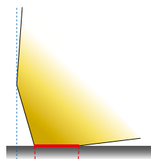
図 ネガティブ刃形による摩耗低減効果 Wear reduction effect of negative edge shape
