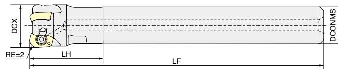
Fig-2 アンダーカット形 Undercut type
