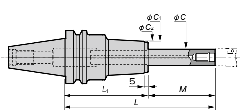
モジュラーミル 取付け部 Dimensions for the Modular Mill mounting
