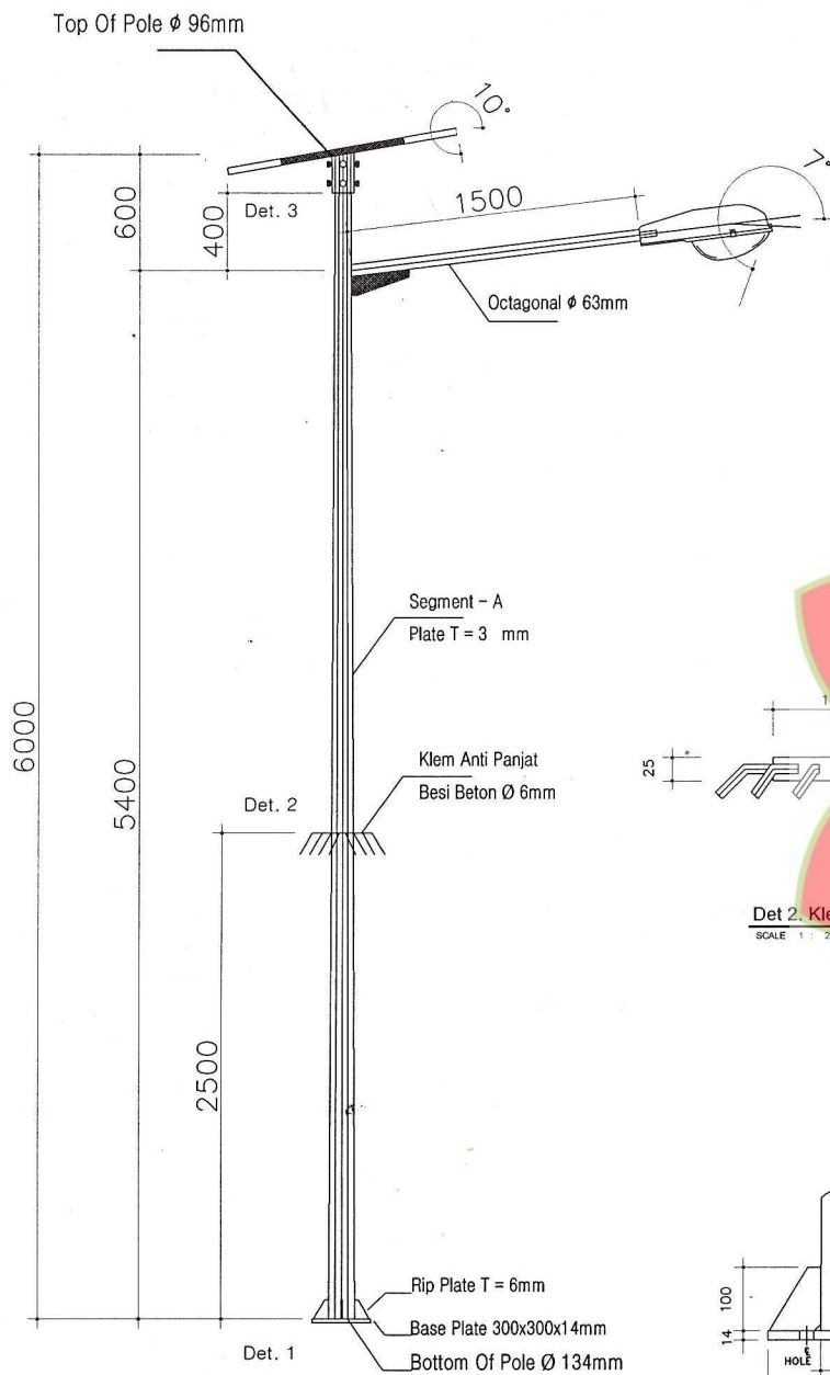
TIANG PJU H-06M SCALE 1 : 100
