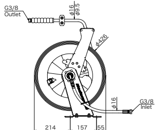
801428 LBM-G, 801237 LBM-16 802238 LBM-30, 801429 LBM-60
